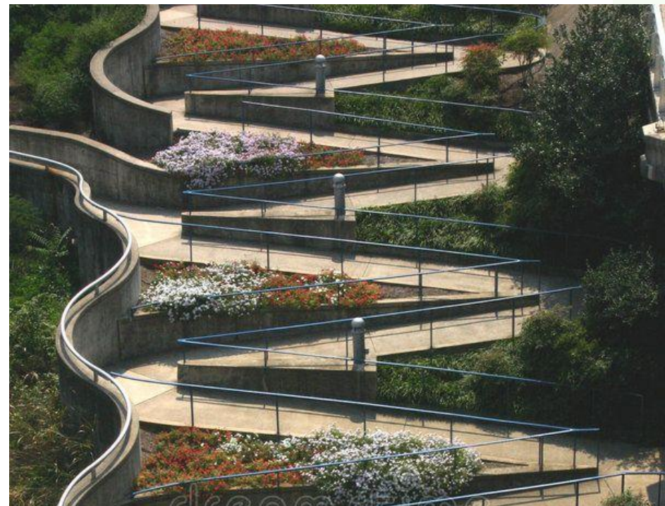
1. NUOVA Rampa accessibilità facile e in autonomia IMMAGINE simile al progetto - Pendenza considerata : 10% - Scala esistente conservata
